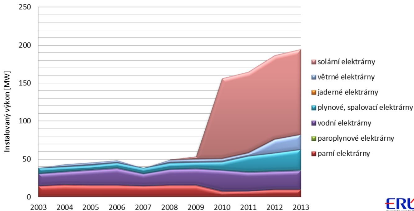
Obrázek č. 4b: Instalovaný výkon zdrojů [MWe], Liberecký kraj, 2013
